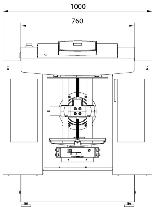
Dimensions BIAX 35
