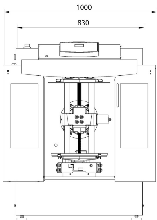
Dimensions BIAX 45
